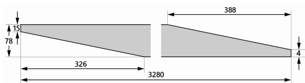
Рисунок 27. Размеры ленты для моделей DS560-W, DS560-WB
