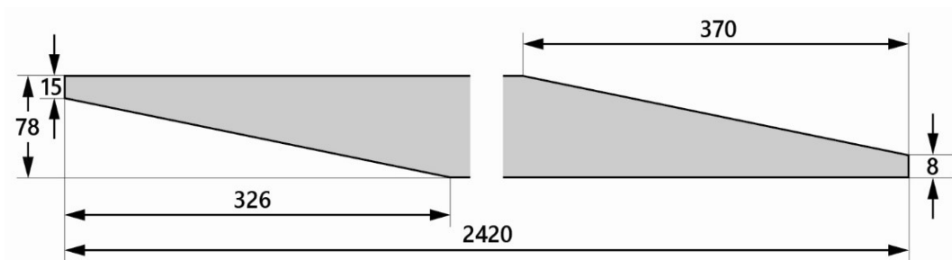
Рисунок 26. Размеры ленты для модели DS410-W
