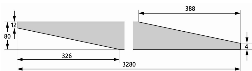
Рисунок 29. Размеры ленты для моделей DS560-W, DS560-WB
